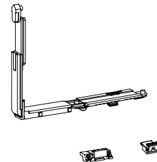
G.053.025 Ponto de Fecho (Adicional horizontal)
