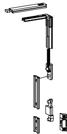
G.053.024 Ponto de Fecho (Adicional vertical)
